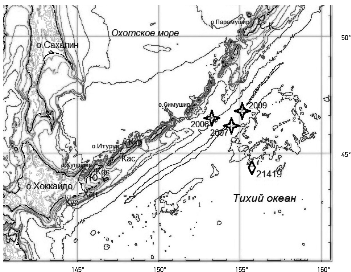
Рис. 1. Расчетная схема численного эксперимента. Звездочками обозначены эпицентры землетрясений, ромбом — положение станции системы DART. На схеме обозначено: Хан — Ханасаки, Кус — Куширо, Ю-К — Южно-Курильск, Кос — бух. Космодемьянская, Кас — зал. Касатка, Кур — Курильск, С-К — Северо-Курильск
